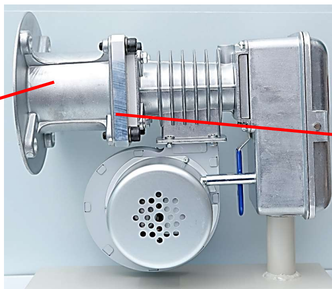
⑦ レジューズプレート付 投光器・受光器
